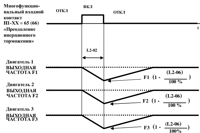
Преодоление инерционного торможения в многодвигательном приводе с общей шиной питания постоянного тока
